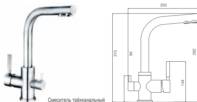
Смеситель трёхканальный
